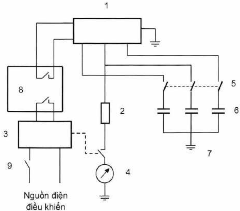
Hình 12. Sơ đồ mô phỏng xác định thời gian cắt khi rò điện 1k \Omega
